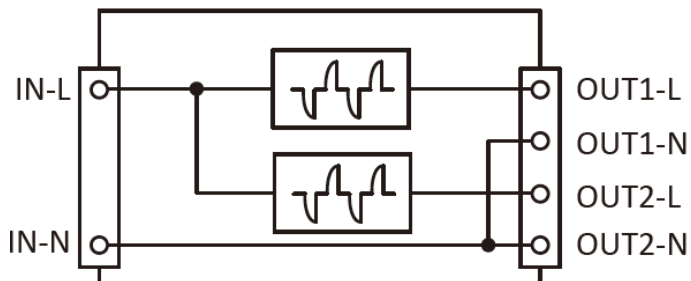
DGTM202 回路図
