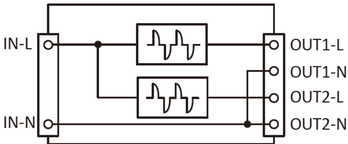
DGLM202 回路図
